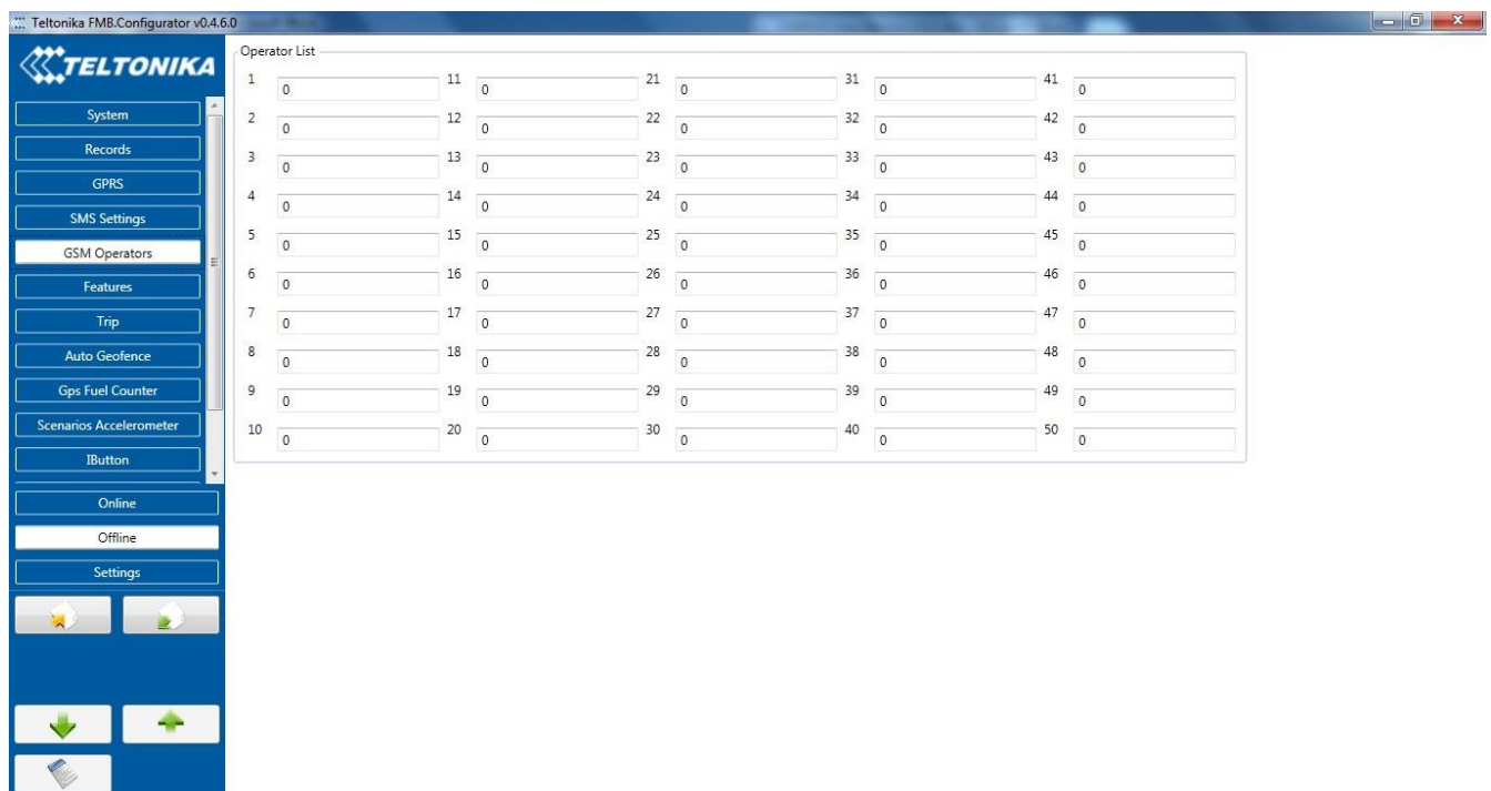
Рис. 15. Конфигурирования списка операторов
