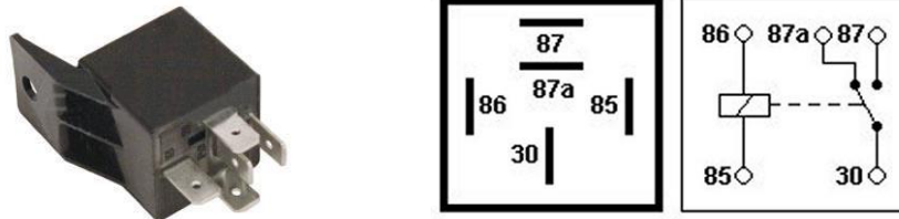
Рис. 8. Схема контактов автомобильного реле
