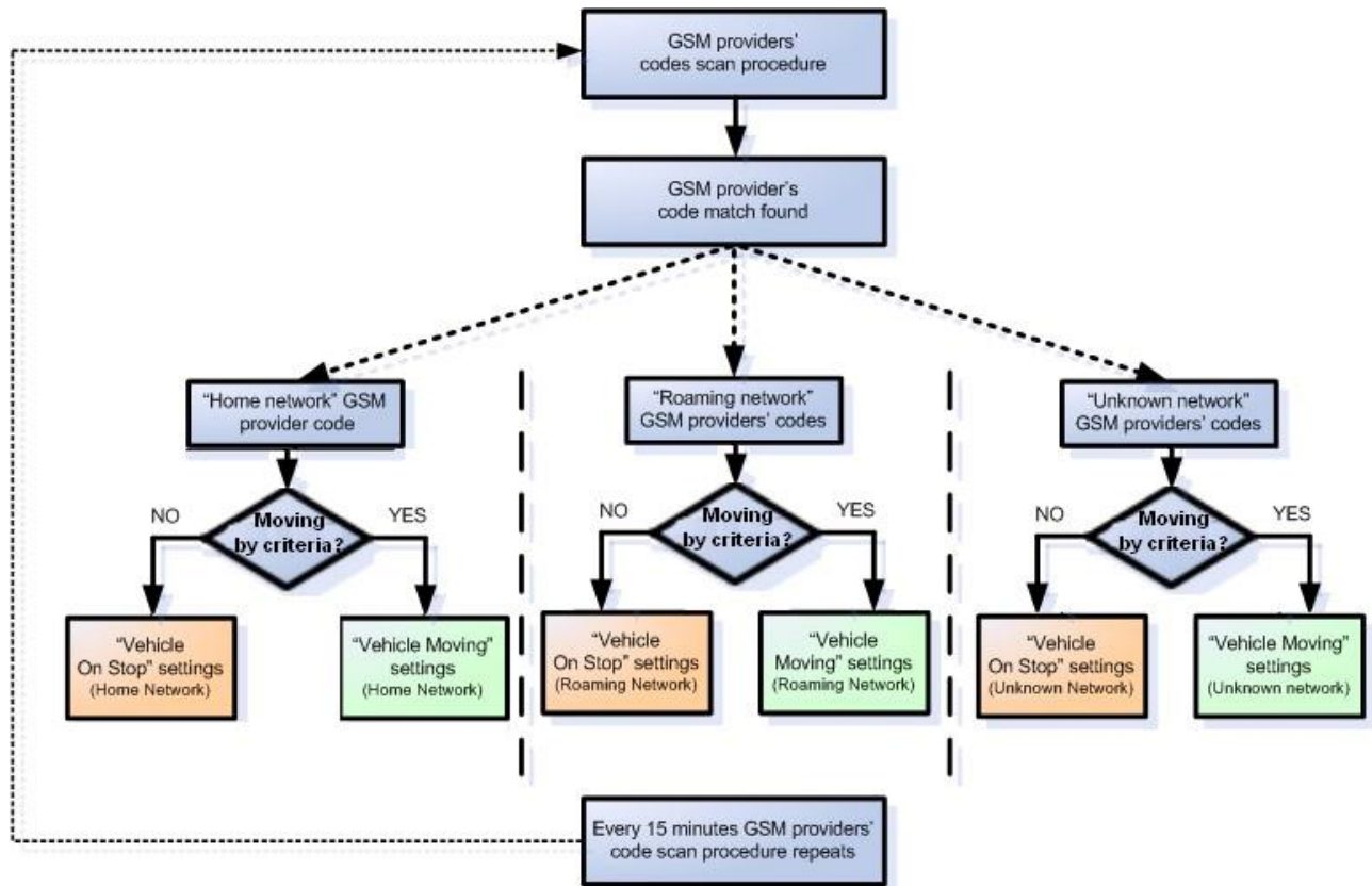
Рис. 16. Выбор режима записи данных
