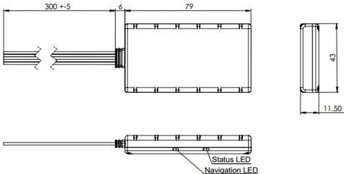
Рисунок 1 Внешний вид и размеры FMB920 (погрешность \pm 2 мм)
